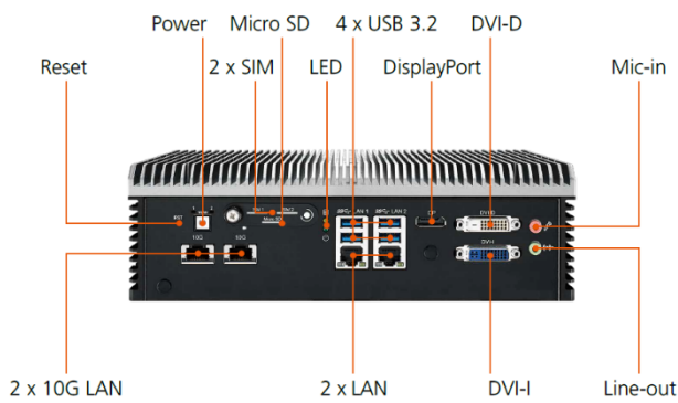
前视图 I/O
